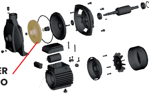
IMPELLER KUNINGAN 402
